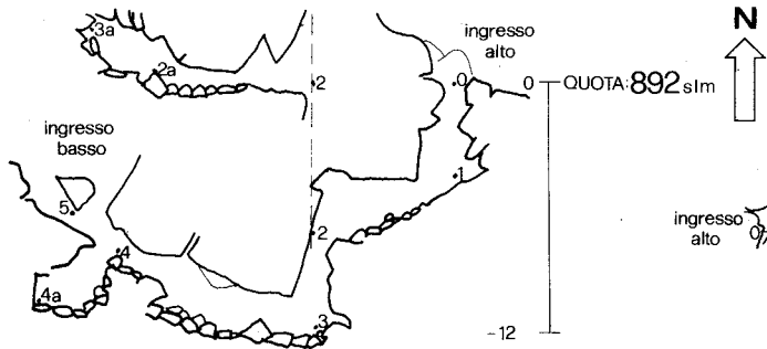
SEZIONE LONGITUDINALE
